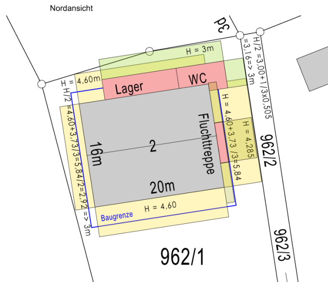
Abb. 7 Geplante Anbauten an das Bestandsgebäude Pfarrstadl mit Darstellung der Abstandsflächen, Böck Architekten 2016, unmaßstäbliche Darstellung
