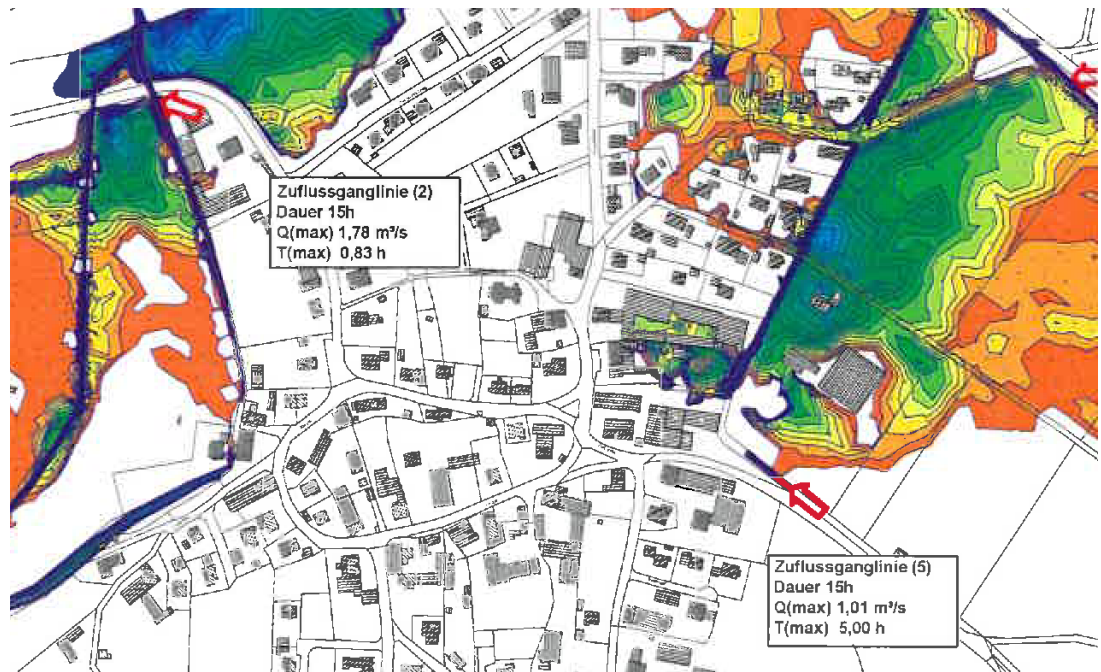
Abb. 5 Auszug aus der Hochwasserfreilegung Überflutungsflächenberechnung, Planeinheit Überflutungsflächen HQ100, im Bereich Untermühlhausen/ Epfenhausen, Ingenieurbüro Wittke Mai 2019.
